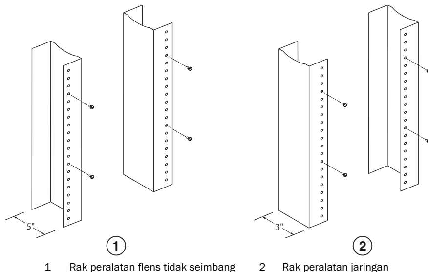
GAMBAR 80 Menentukan posisi baut pemasangan pada tempat rak
