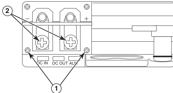
1 Baut yang menahan penutup plastik 2 Baut yang menahan tab daya
