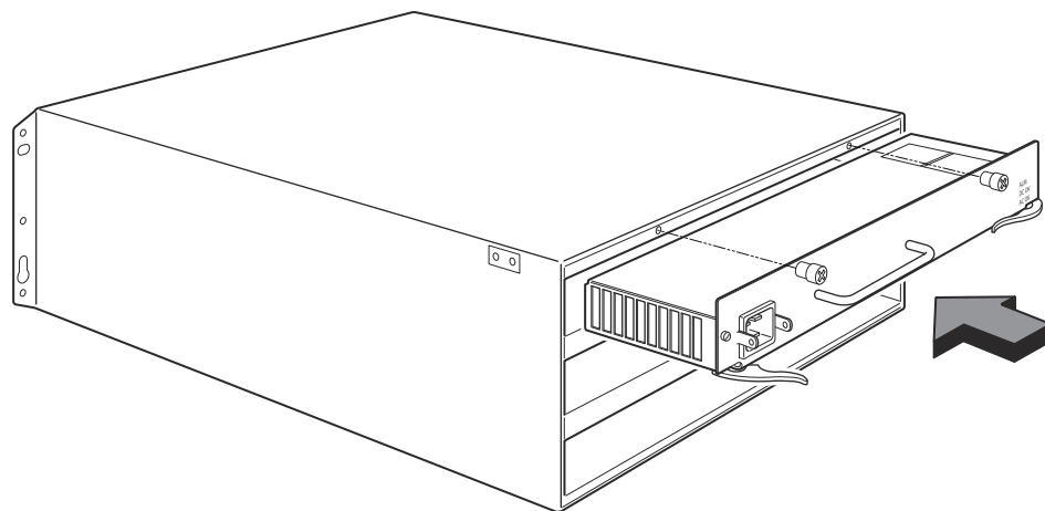
GAMBAR 85 Memasang catu daya di dalam sasis 4 slot
