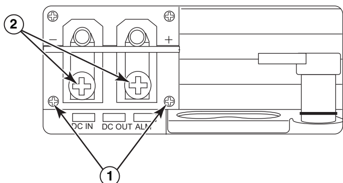
图 14 适用于 8 插槽和 16 插槽机箱的直流电源设备
