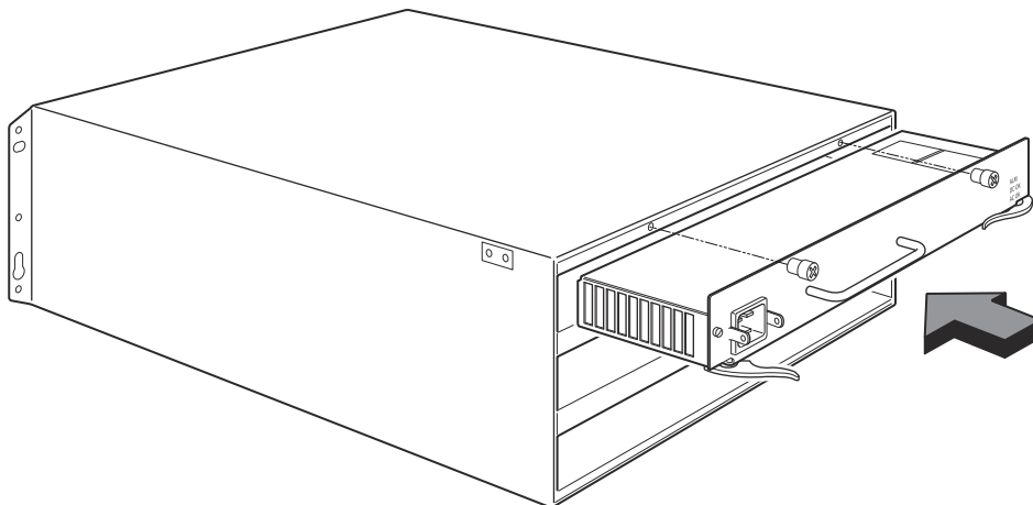
ABBILDUNG 70 Netzteilinstallation in einem Gehäuse mit 4 Einschüben
