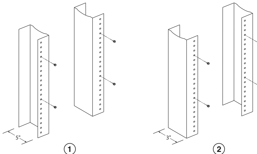
FIGURE 50 Positionnement des vis de montage dans les supports verticaux de rack
